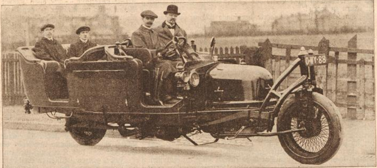
Ein zweirädriges Automobil. (Mit Text.)
