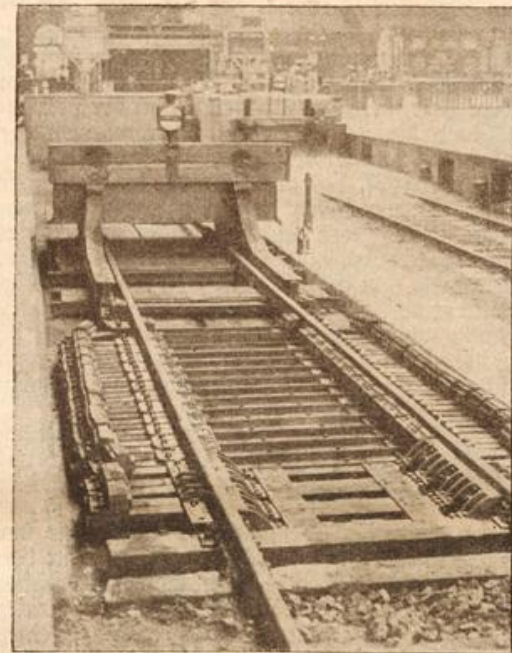
Ein neuer Bremspressblock mit Schlepptrost auf dem Stettiner Bahnhof in Berlin.
