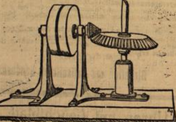
Abb. 1. Antrieb mit Vorgelege.
