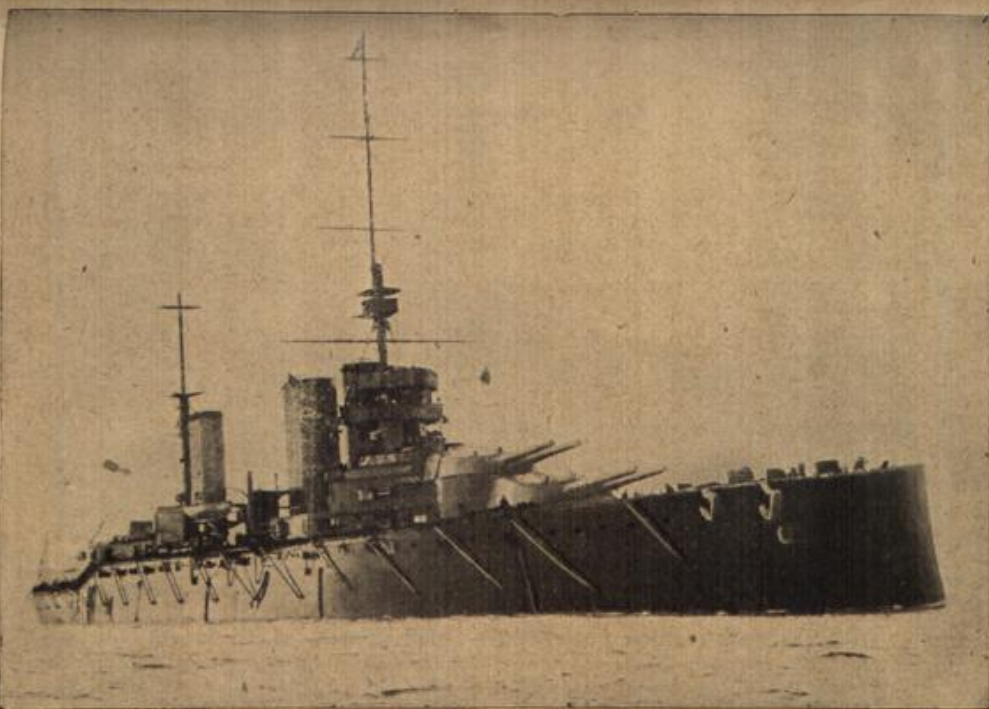
Der englische Schlachtkreuzer „Queen Mary“, welcher im Kampfe vernichtet wurde. Stapellauf 1912, Wasserverdrängung 30 000 Tonnen.
