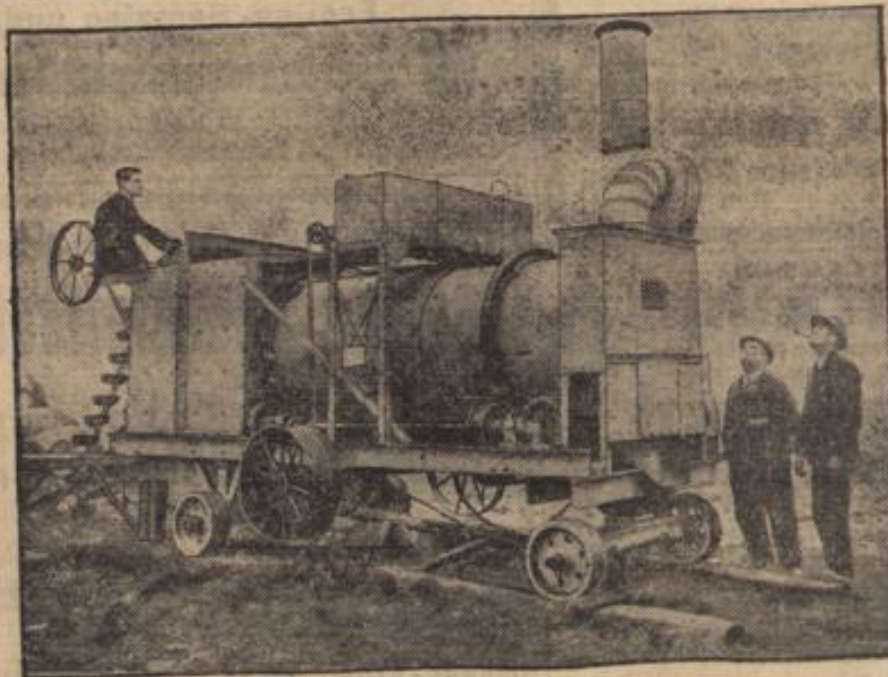
Die Betons-Lokomotive.
