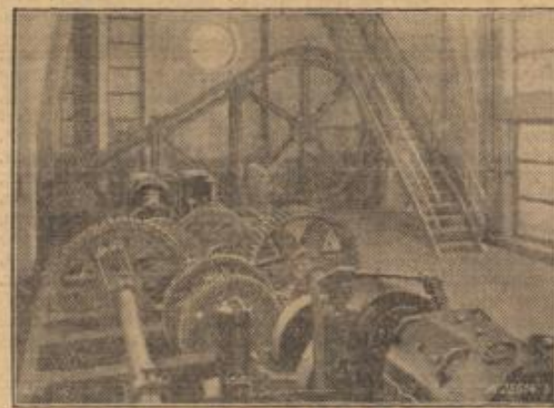
Blick in eines der Maschinenhäuser der Nordischen Schleuse Bremerhaven: Torantriebswinde.
