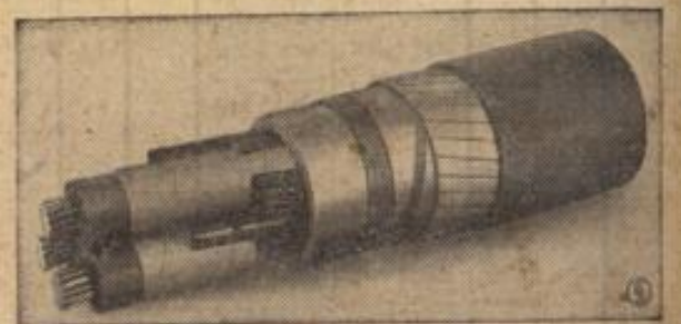
Aufbau des Siemens-Kabels.
