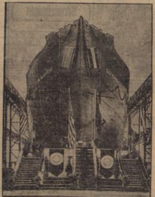
Stapellauf eines Riesen-Motortankschiffes in Kiel. Das Motorschiff „Geo W. Mc. Knight“ kurz vor dem Stapellauf. Das Motorschiff, das 16 200 Tonnen groß ist, gehört zu einer Serie von 6 Schiffen, die für Rech-nung der amerikanischen Ölgesellschaft auf deutschen Werften zur Zeit gebaut werden.
