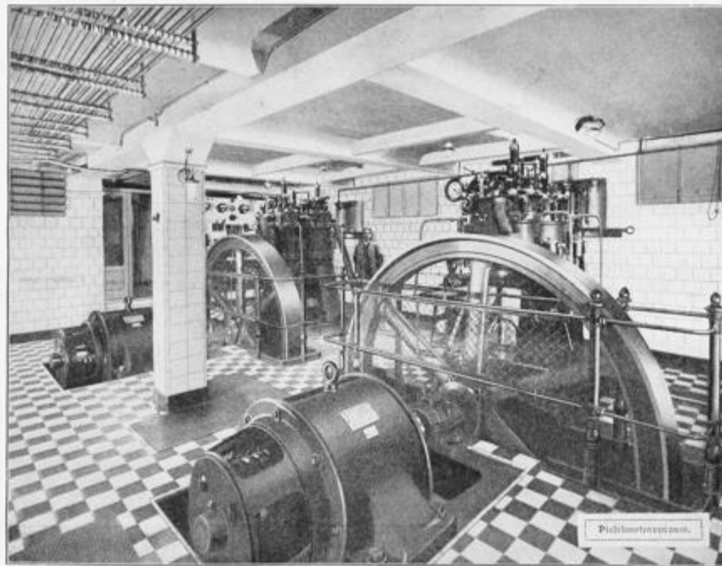
Dieselmotorenraum.
