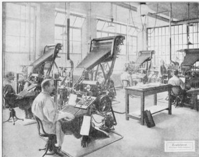
Teil des Linotype-Setzmaschinenraums.
