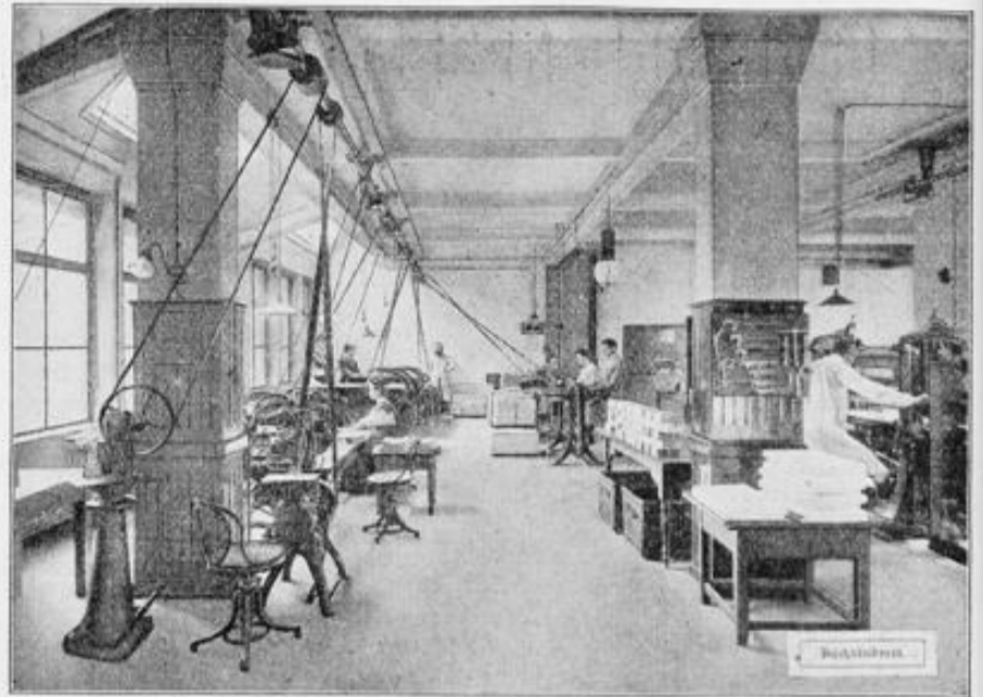
Teil der Buchbinderei.
