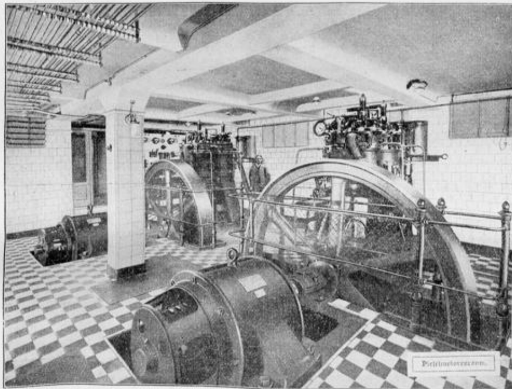
Dieselmotorenraum.
