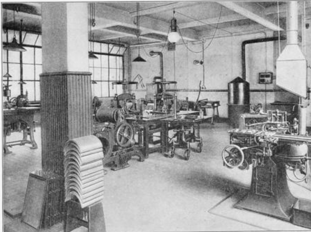
Teil der Stereotypie mit Monotype-Gießmaschine.
